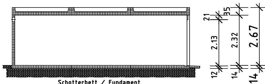
Schnitt
