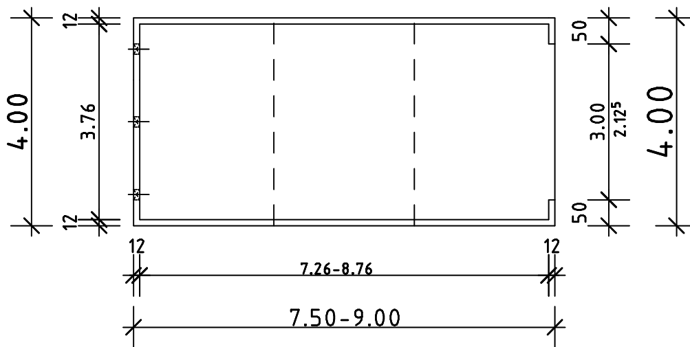
Grundriss
