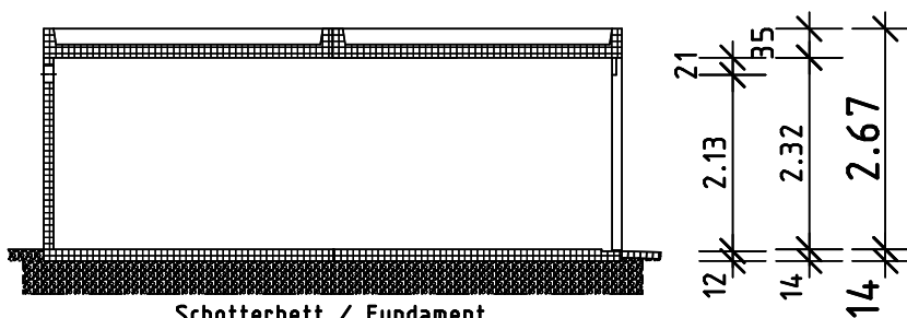
Schnitt
