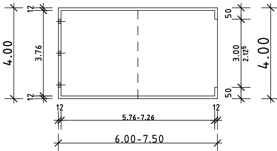
Grundriss
